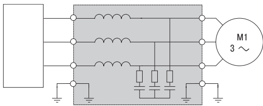
Фильтр dU/dt
